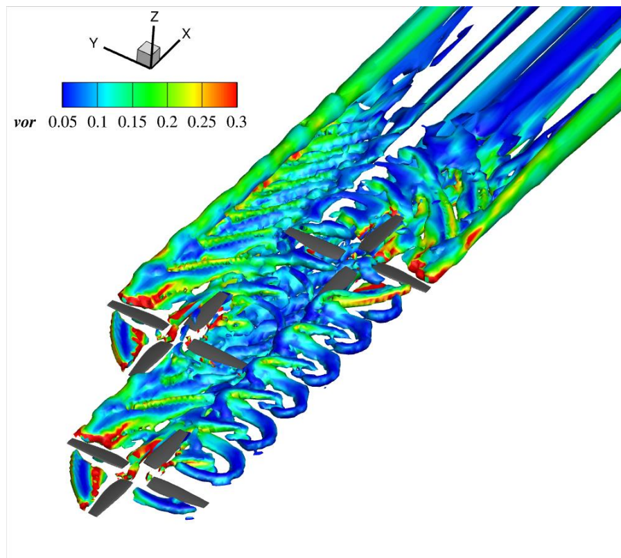
図 1: マルチロータ周りの複雑な翼端渦流れ場の様子
