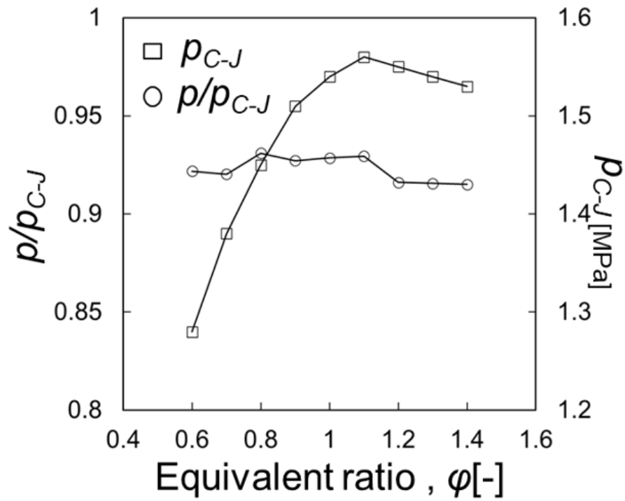
図 3: 等量比と爆轟波背後圧力の関係
