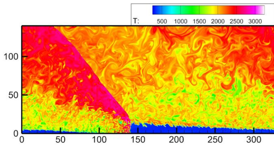
図 2: 燃焼器内部を伝播する爆轟波の温度分布
