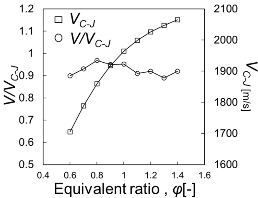
図 4: 等量比と爆轟波背後温度の関係
