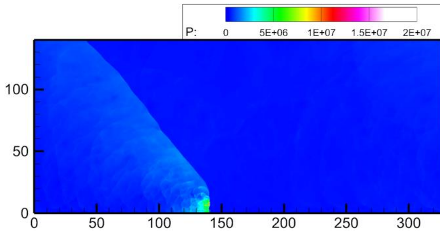
図 1: 燃焼器内部を伝播する爆轟波の圧力分布
