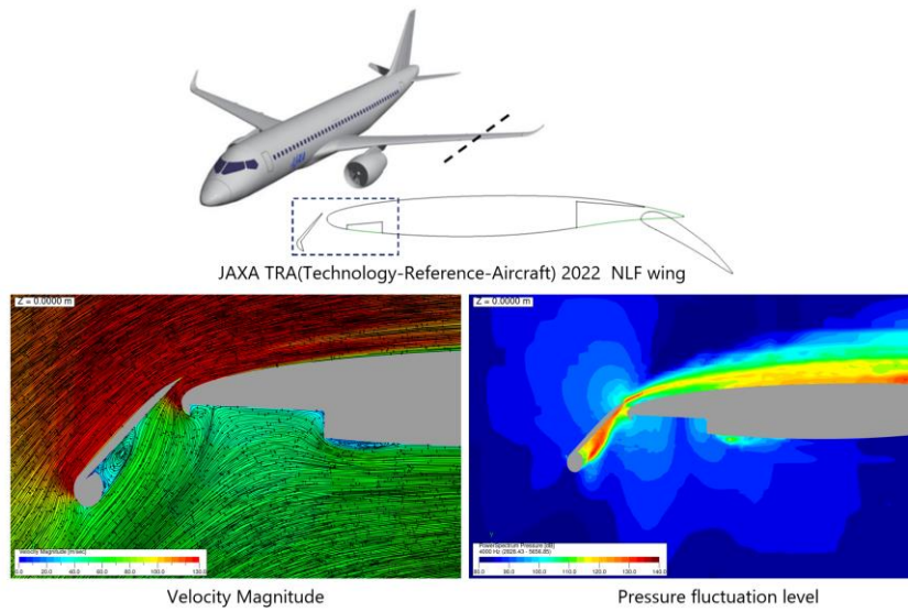
図 1: クルーガーフラップの騒音評価解析
