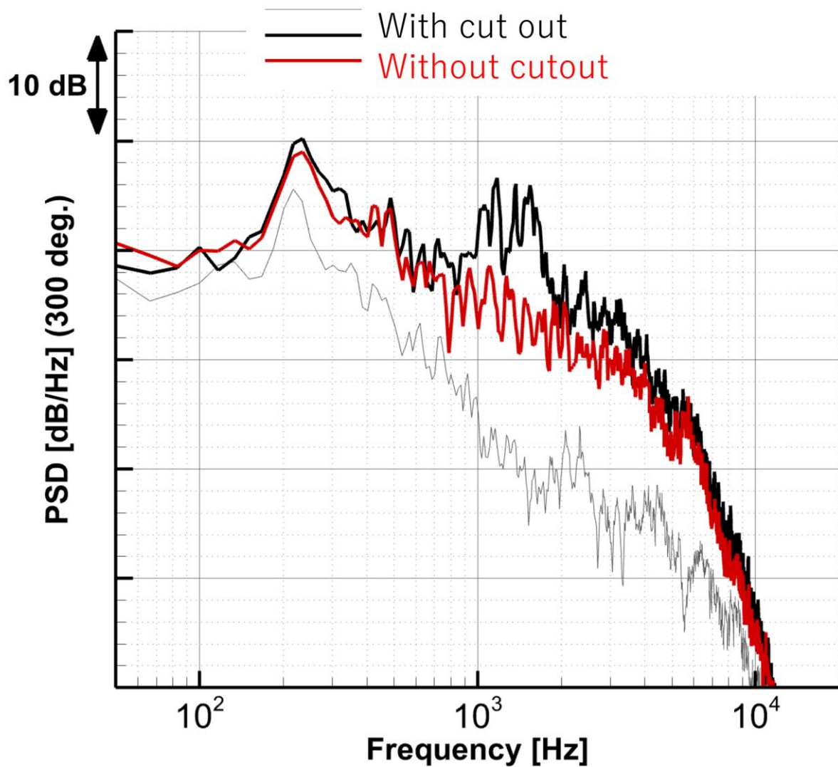
図 2: スラット支持展開機構のカットアウト有無による騒音レベルの変化
