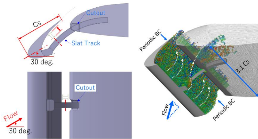
図1: スラット支持展開機構から生じる騒音評価に用いた解析形状
