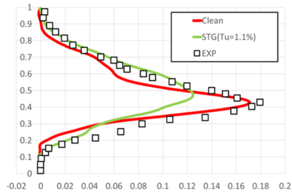
図 2: 翼後流の全圧損失分布における実験値との比較
