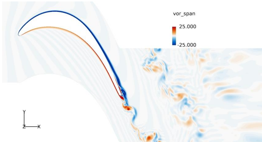
図 1: LES による直線翼列の解析結果(渦度分布)
