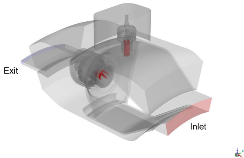
図 1: 燃焼解析用計算領域
