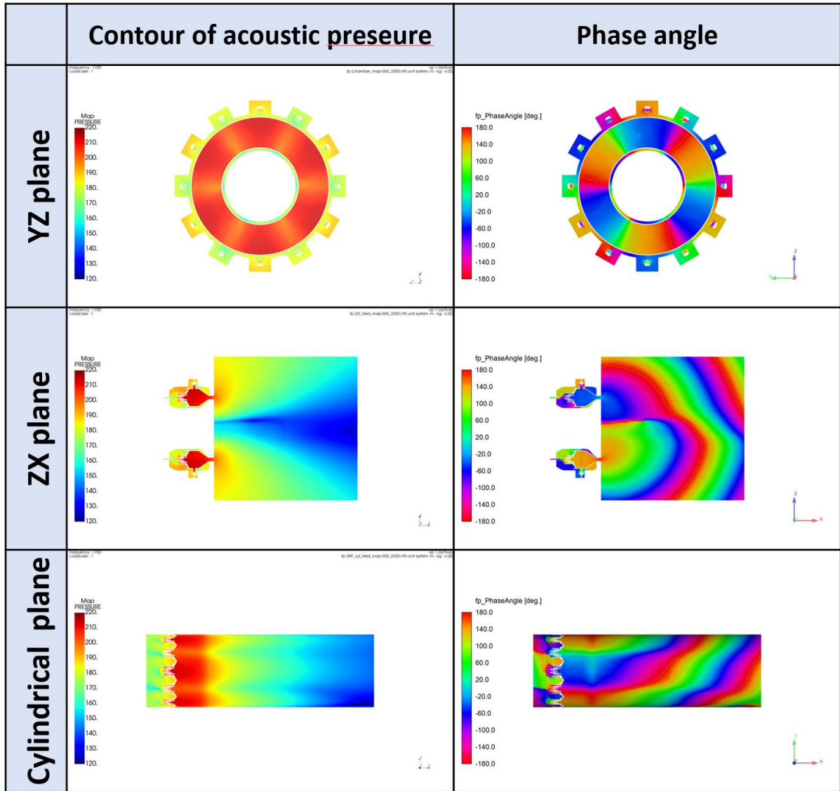
図 3: 各断面上の音圧・位相コンター
