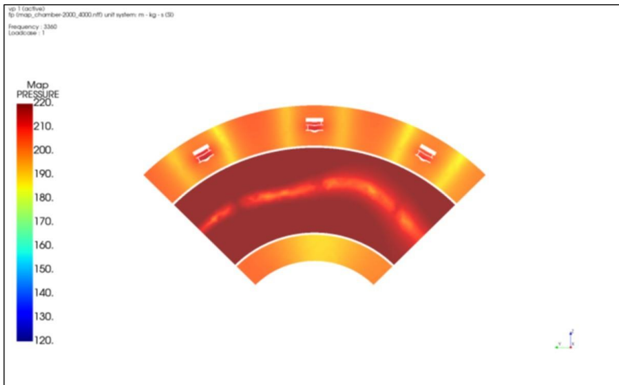
図 4: 音圧コンター
