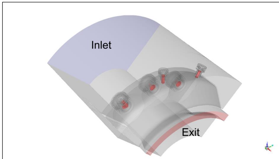
図 1: 燃焼解析用計算格子
