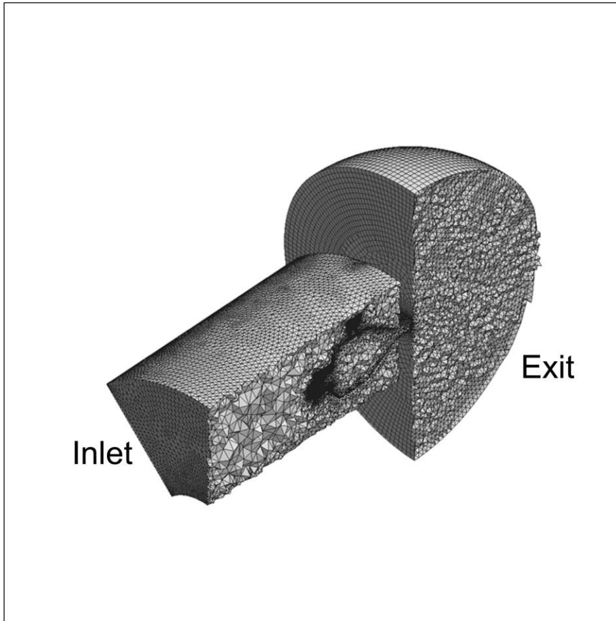
図 3: 音響解析用計算格子
