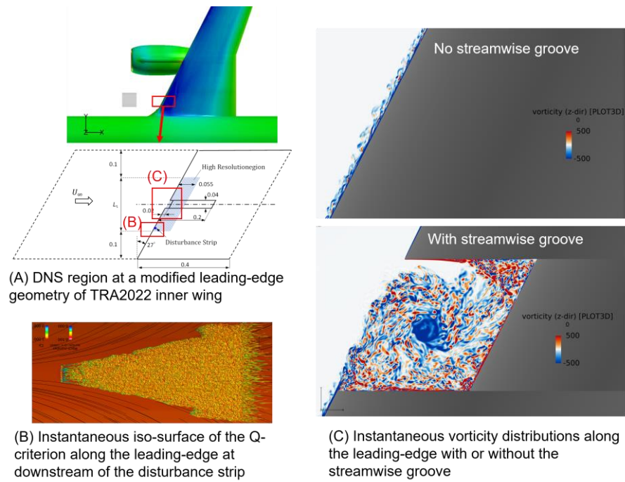
図 1: TRA2022 主翼の付着線汚染による境界層遷移を防止する空力デバイス streamwise groove 周りの流れ
