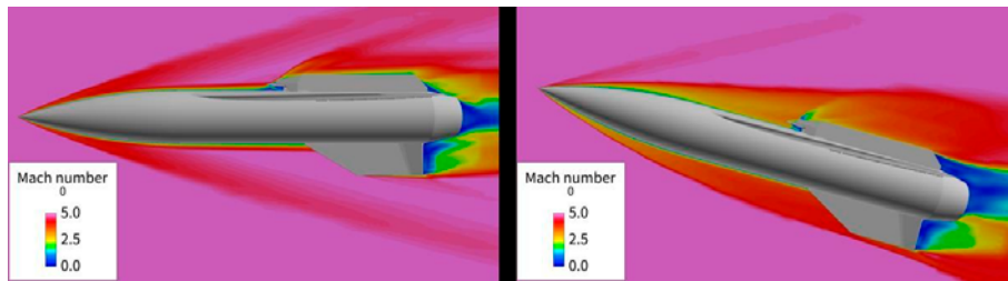
図 2: 極超音速統合制御実験機(オジャイブノーズ)のマッハ数分布(マッハ 5, 迎角: 0deg, -15deg)
