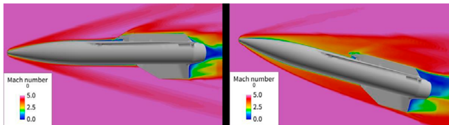
図 3: 極超音速統合制御実験機(パラボリックノーズ)のマッハ数分布(マッハ 5, 迎角: 0deg, -15deg)
