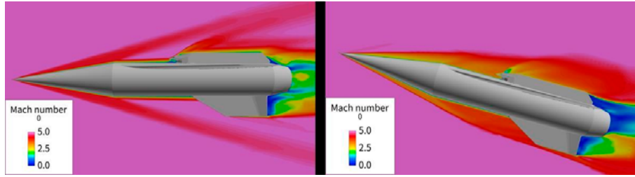
図 1: 極超音速統合制御実験機(円錐ノーズ)のマッハ数分布(マッハ 5, 迎角: 0deg, -15deg)
