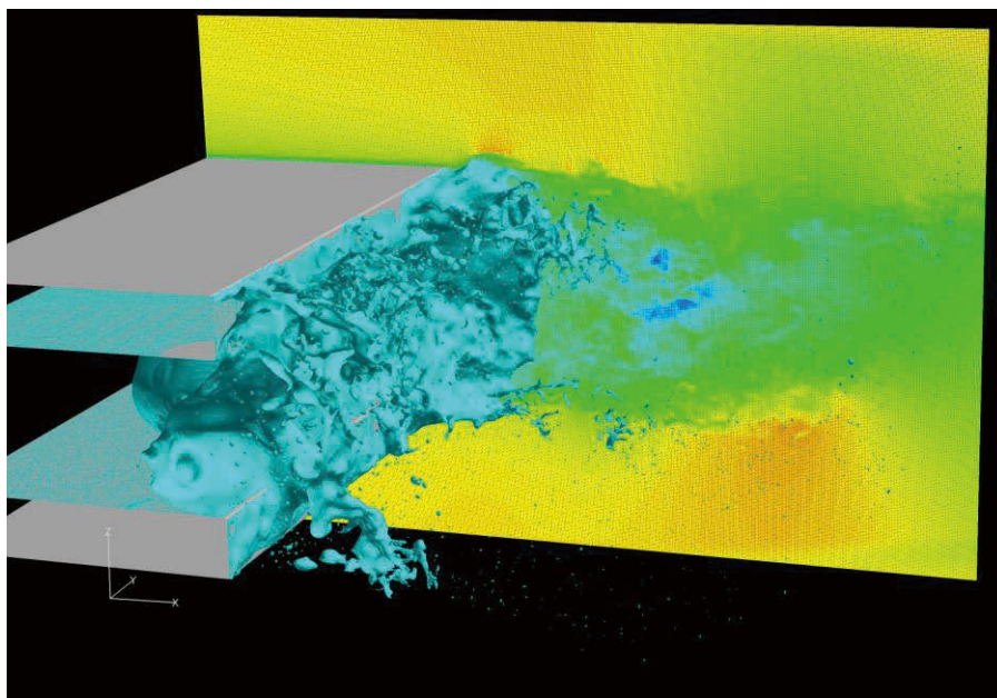
図 1: 平面液膜式噴射弁における燃料微粒化
