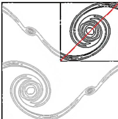
図 1: primary vortex のプロファイル計測位置
