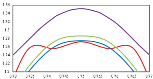
図 3: primary vortex のプロファイル(ピーク拡大図)
