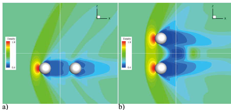
図 1: 超音速流れにおける 2 つの微粒子の干渉流れ; a) 直列, b) 並列
