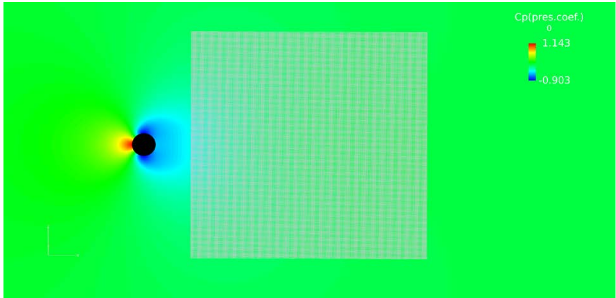
図1 円柱周りの流れ場(グリッド部分を学習データとして使用)
