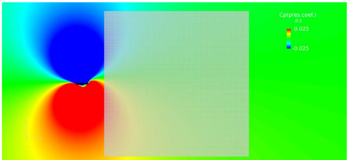
図2 翼周りの流れ場(グリッド部分を学習データとして使用)
