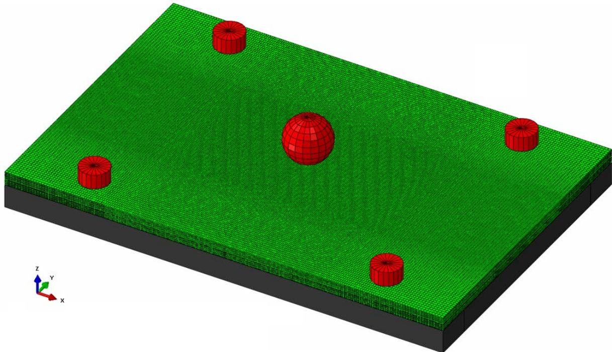
図1 CFRP に対する低速衝撃シミュレーションモデルの外観
