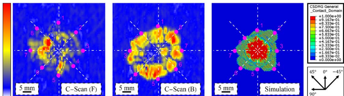
図2 シミュレーションによって予測された損傷と実験によって観測された損傷の比較
