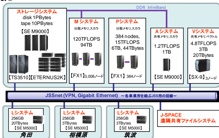
▲JSS (JAXA Supercomputer System) システム構成図
